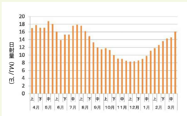
図1 全日射量の推移(名古屋・平年値)
