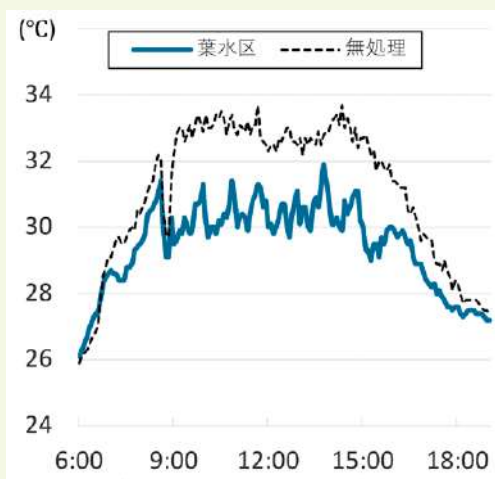
▲図1 日中葉水による典型的な温度推移
