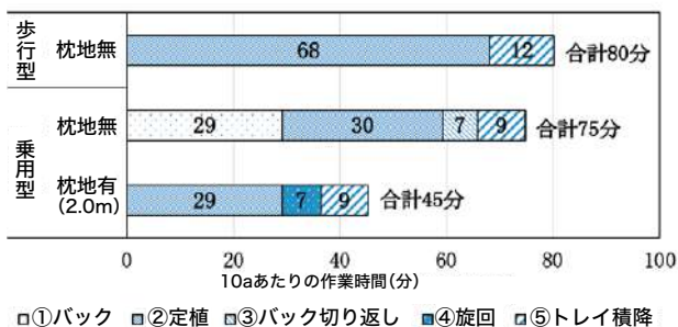
▲図1 乗用・歩行型移植機の作業時間
