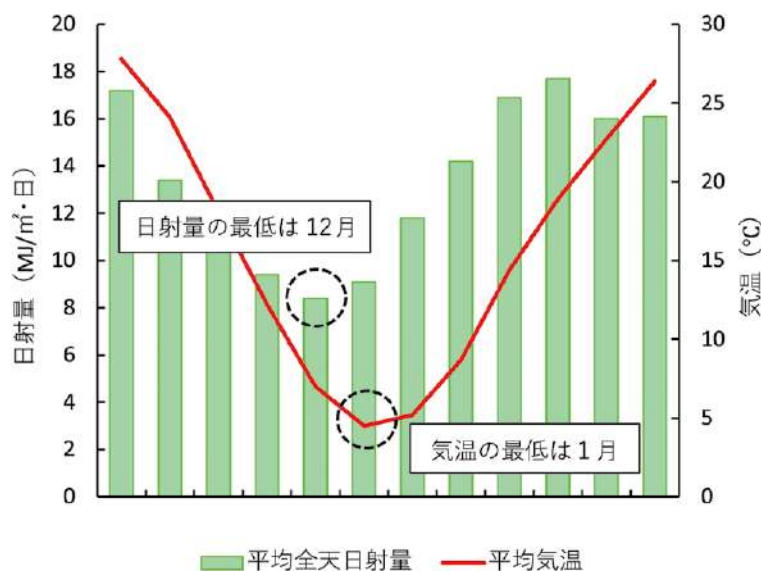
図1 日射量と気温の変化(名古屋平年値)
