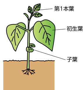
図3 葉の名称
